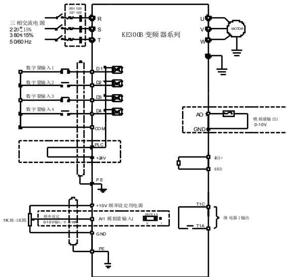
图 3-3 KE300B 系列变频器接线图
