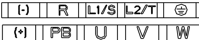
图 3-7 主回路端子图 (KE300B 系列单相 220V-0.4~2.2kW/380V-0.75-4kW)
