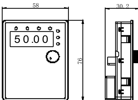
KE300X 系列单相/三相 220V 0.4~1.5kW
