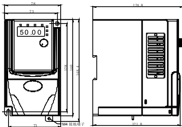
KE300X 系列单相/三相 220V 0.4~1.5kW
