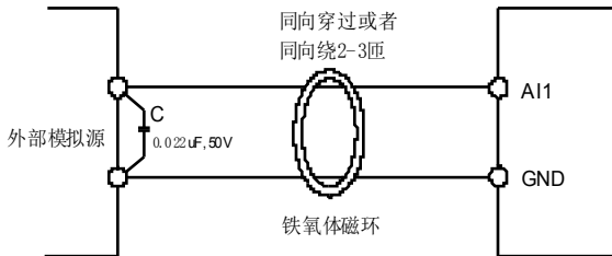
图 3-16 模拟量输入端子处理接线图
