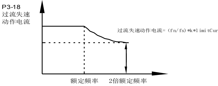
倍速过流失速动作示意图
