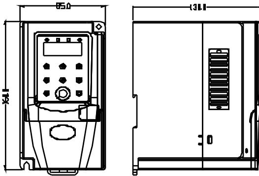
KE300B 系列 单相 220V 0.4~2.2kW 变频器尺寸
