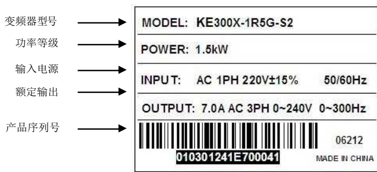
图 2-2 KE300X 铭牌说明
