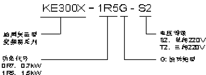
图 2-1 KE300X 型号说明
