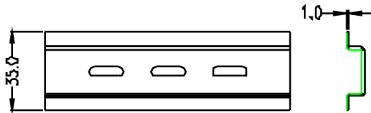
安装导轨尺寸图
